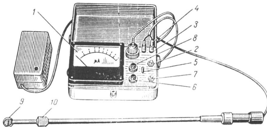
Мал. 5. Електротермоанемометр
